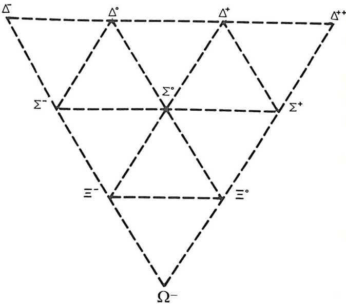
the baryon decuplet
