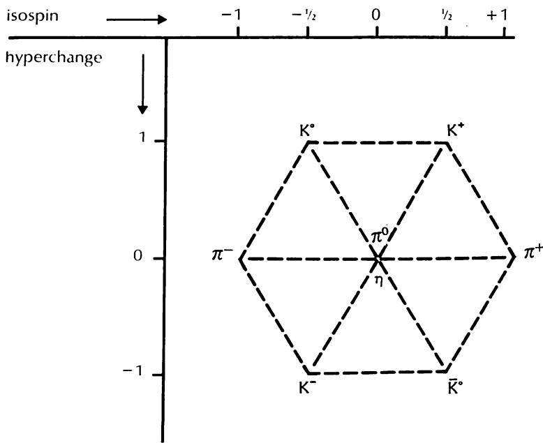
the meson octet
